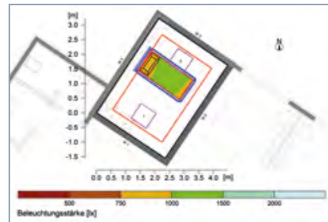
Lichtplanung 1-Bett-Zimmer, Meßfläche auf dem Bett
